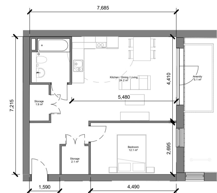
1B2P_E 1 : 100
