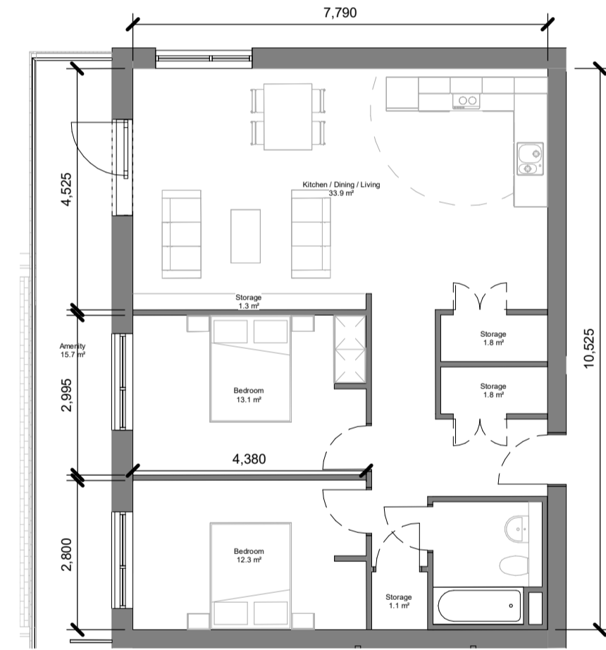
2B4P_M 1 : 100
